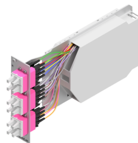
Spleiß - Einschubmodul für bis zu 24 Fasern
