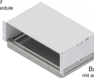
Baugruppenträger 3HE 19" für bis zu 12 Einschubmodule
